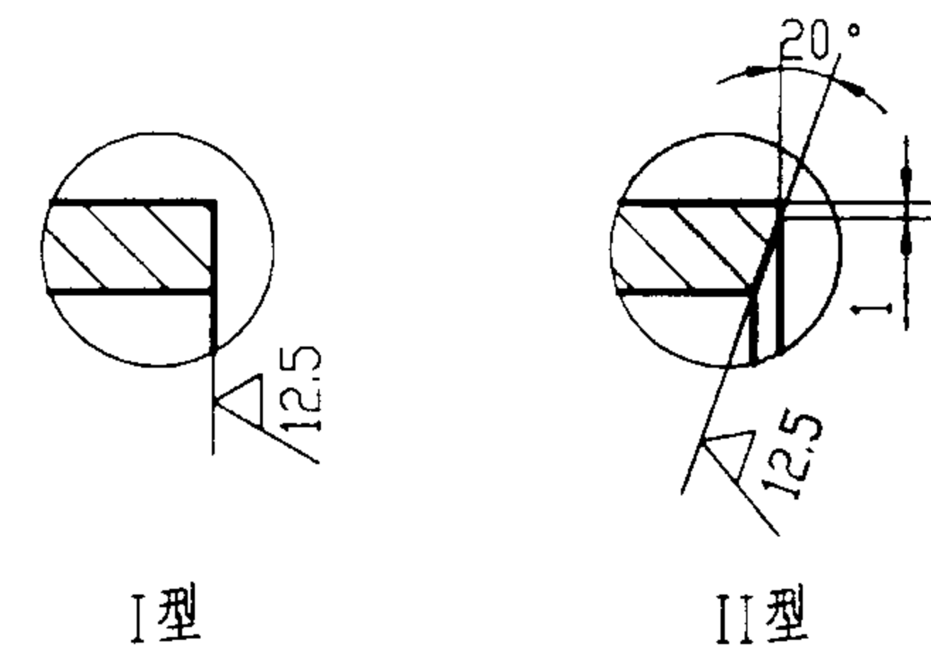
短管结构
